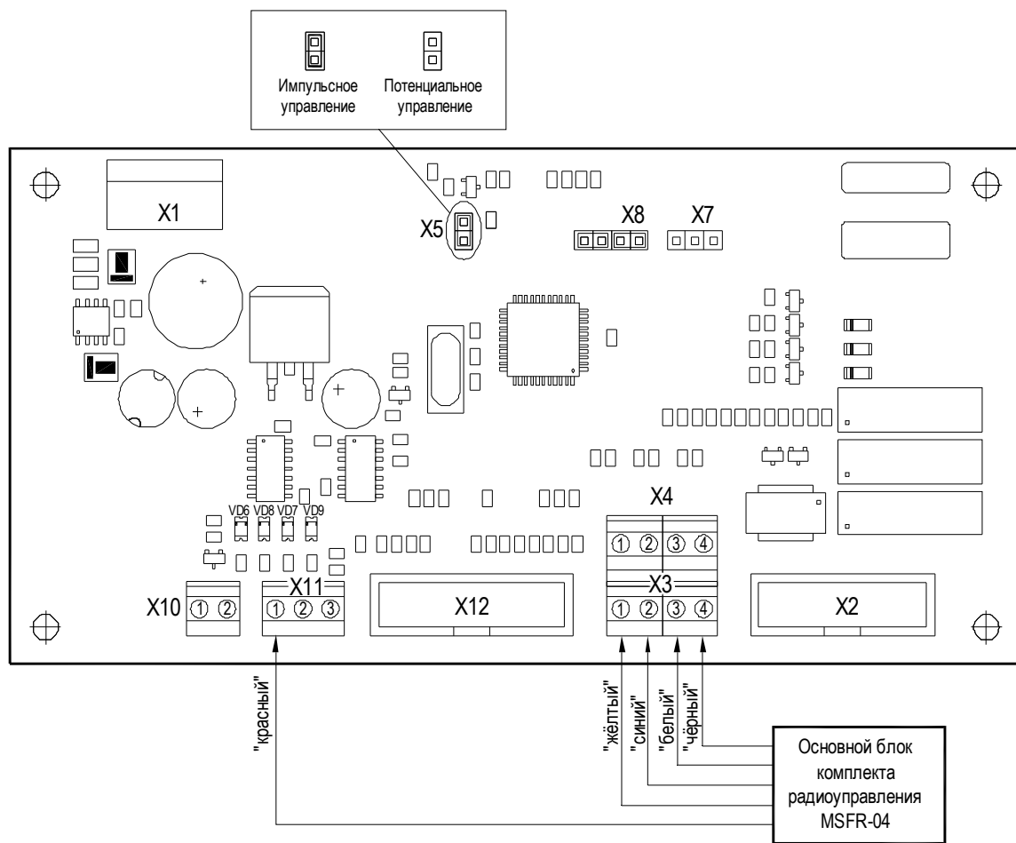
Рис. 9. – Схема подключения устройства радиуправления MSRF-04 к модулю процессорному
