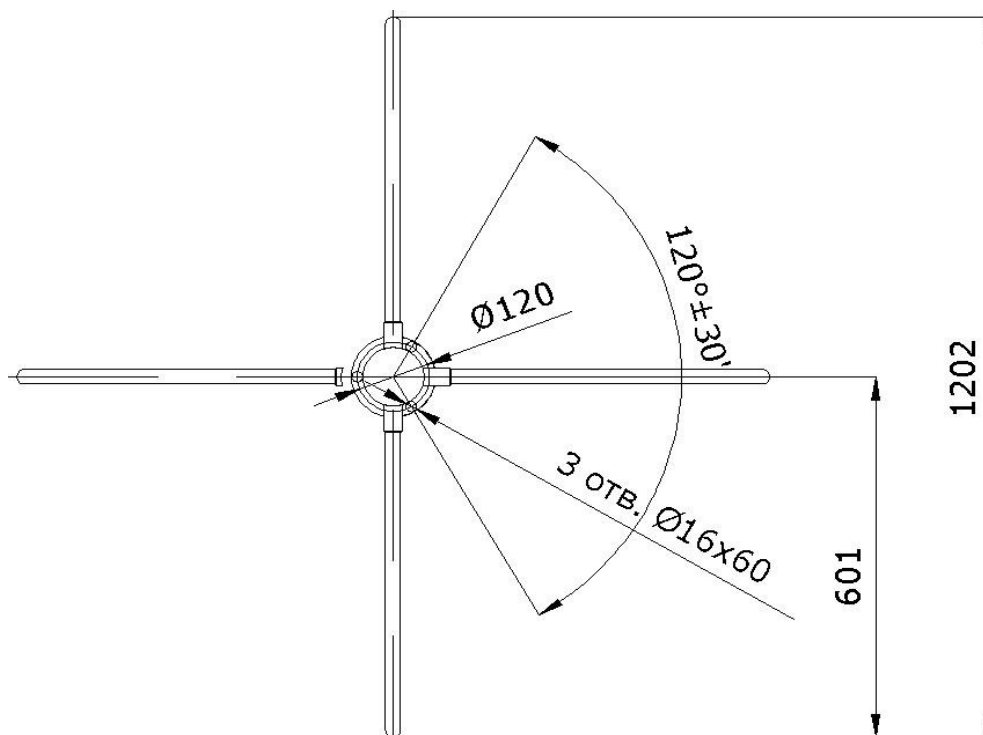
Рис. 6. Схема разметки для монтажа турникета
