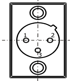
Рис. 4. Назначение контактов разъемов блока управления
