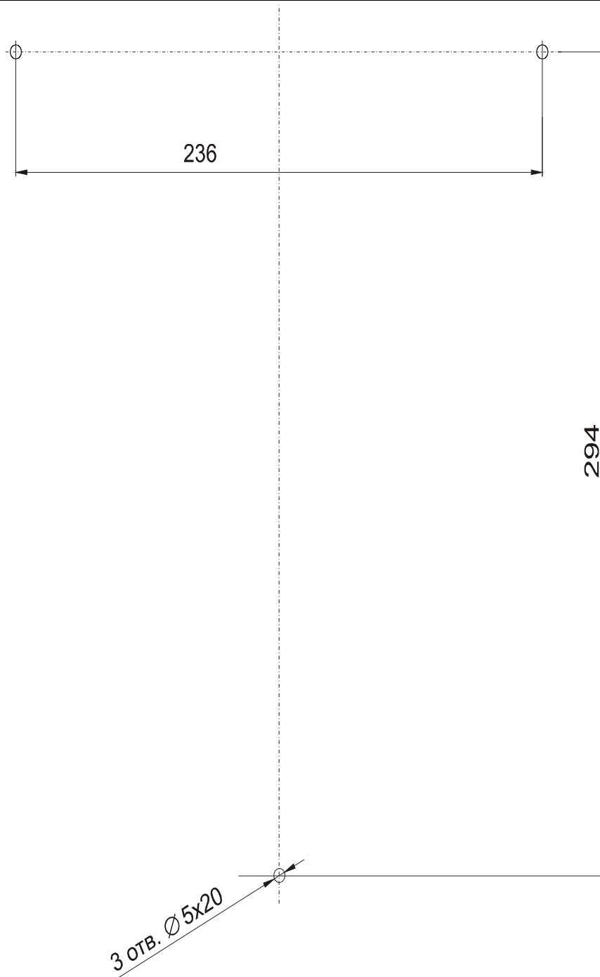
Рис. 7. Разметка отверстий для установки блока управления
