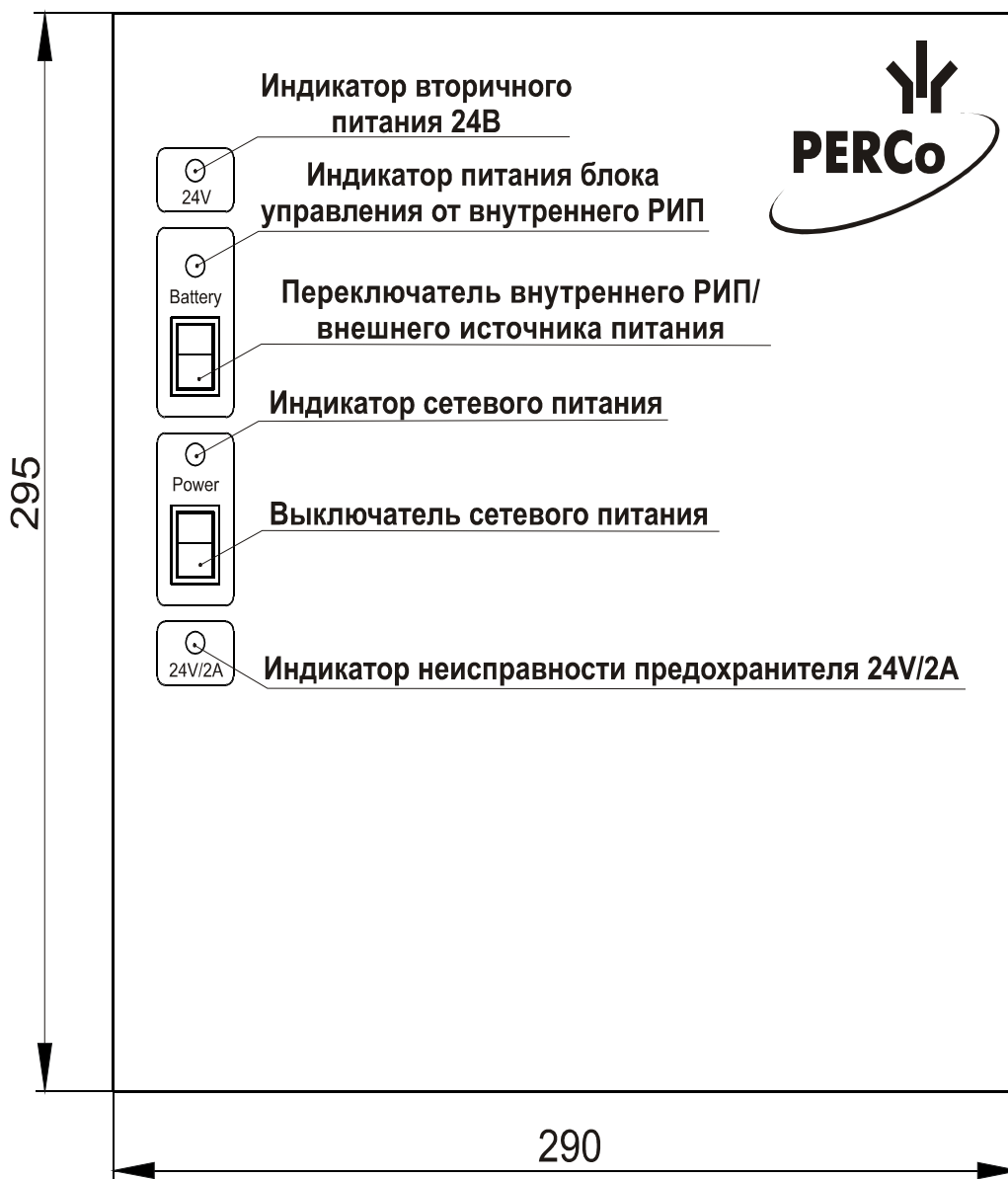
Рис. 3. Блок управления
